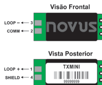
Fig. 3 – Saída 4-20 mA (sem M12)
