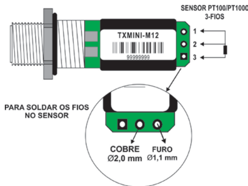
Fig. 5 – Entrada Pt100 / Pt1000 3 fios
