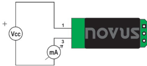
Fig. 4 – Diagrama de Conexão do TxMini / TxMini-M12
