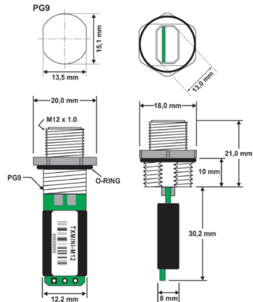
Fig. 2 – Dimensões do transmissor
