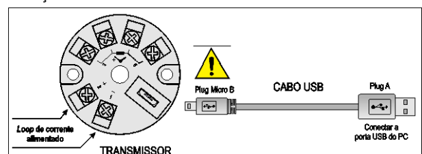
Fig. 1 – Conexão do cabo USB
