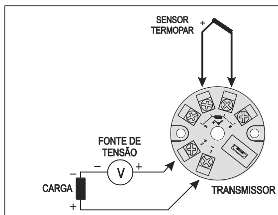
Fig. 9 – Conexões elétricas do transmissor (Termopar)
