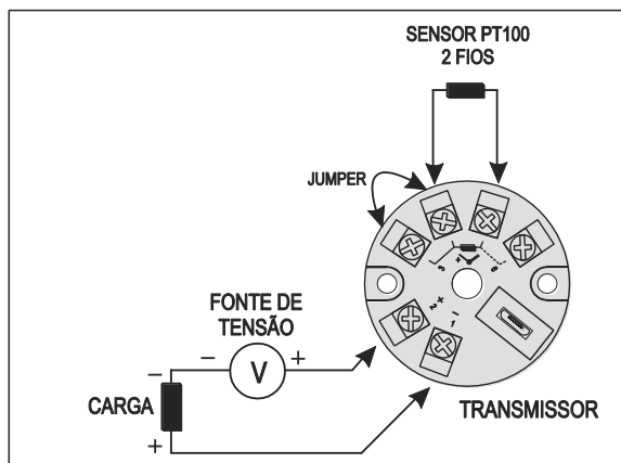
Fig. 5 – Conexões elétricas do transmissor (Pt100 2 fios)
