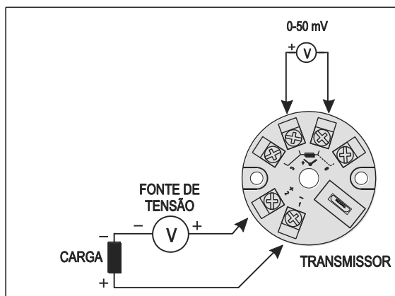
Fig. 10 – Conexões elétricas do transmissor (0-50 mV)
