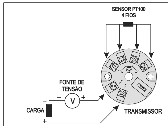
Fig. 7 – Conexões elétricas do transmissor (Pt100 4 fios)
