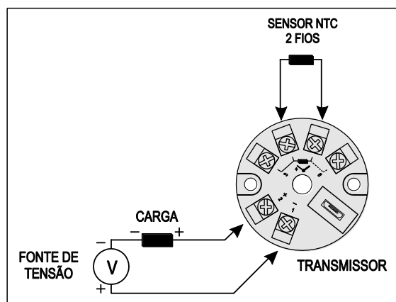
Fig. 8 – Conexões elétricas do transmissor (NTC 2 fios)
