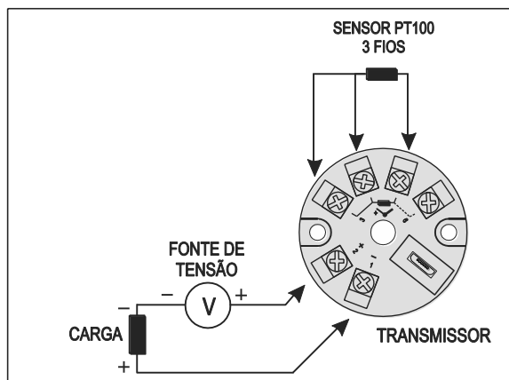
Fig. 6 – Conexões elétricas do transmissor (Pt100 3 fios)
