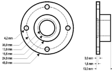
Fig. 06 - Flange para a fixação do modelo RHT/DM.
