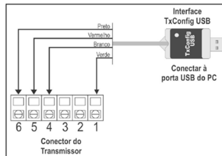
Fig. 03 – Conexões da Interface TxConfig USB
