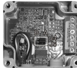
Fig. 09 - Localização dos Jumpers J4 e J5 no interior do transmissor
