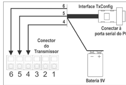
Fig. 02 – Conexões da Interface TxConfig modelo RS232
