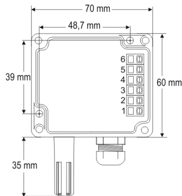
Fig. 08 - Furos de fixação e medidas do modelo RHT/WM.
