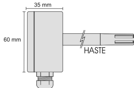
Fig. 07 - Dimensões do modelo RHT/DM.
