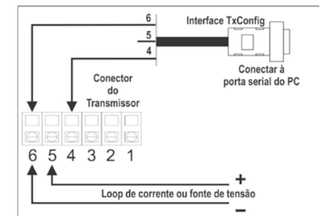
Fig. 05 – Conexões da Interface TxConfig – Alimentação pelo loop
