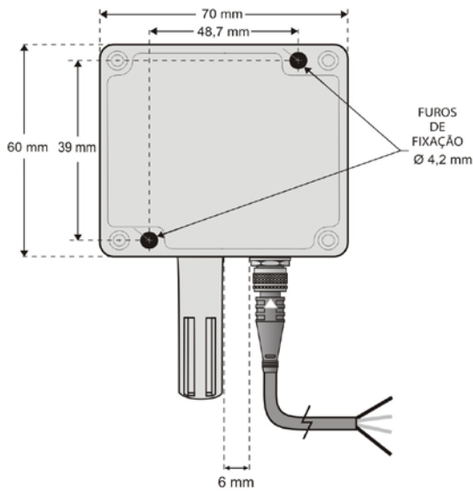
Fig. 4 - Furos de fixação e medidas do RHT-Air
