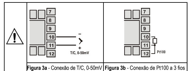
Figura 3a - Conexão de T/C, 0-50mV
