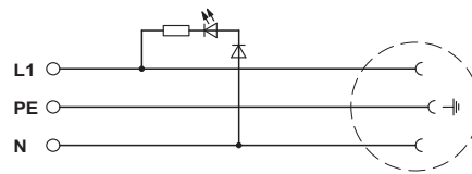
Diagrama de circuitos
