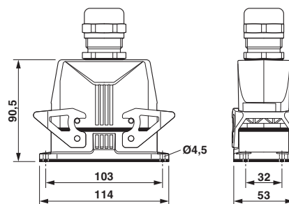
Imagem dimensional
