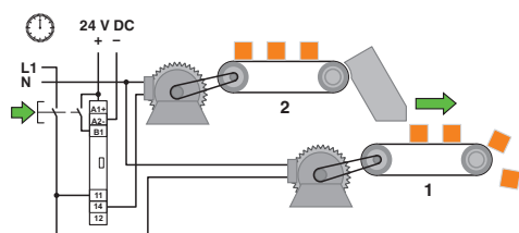
Esteira transportador 1 inicia imediatamente
