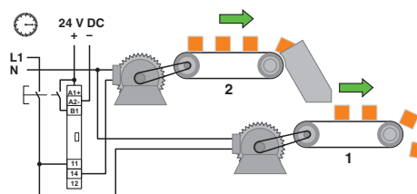
Esteira transportadora 2 inicia com retardo
