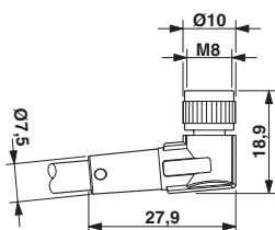
Desenho de medidas
