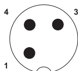
Conector Polbild M12, 3 pólos, codificação A, vista lado do suporte
